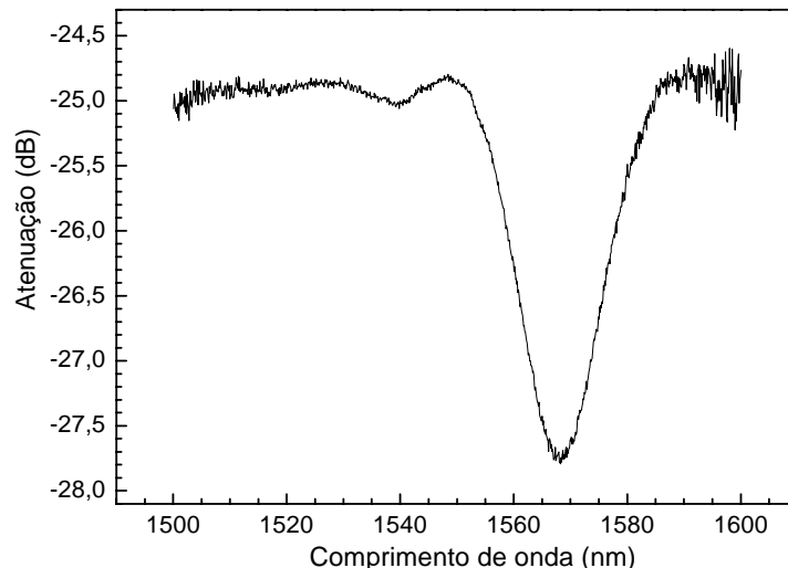
Figura 17 – Razão dos espectros do sinal da rede (LPG1b) e do sinal do LED.
