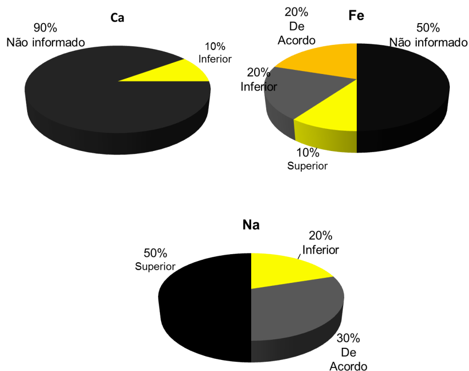
Figura 4. - Comparação das concentrações obtidas para Ca, Fe e Na em amostras de achocolatado em pó com os valores informados nos rótulos das embalagens. Considerados os valores médios obtidos.
