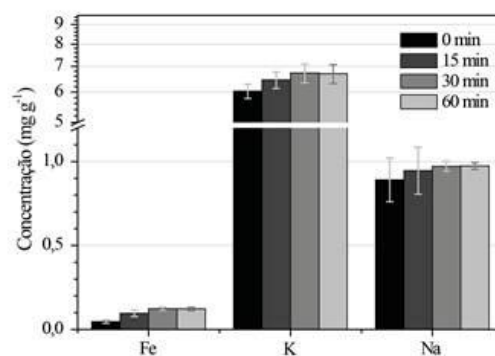
Figura 2. Influência do tempo de extração sob a concentração de Fe, K e Na em achocolatado empó. Solução extratora de \text{HNO}_3 50% v.v -1 e temperatura de extração 50 \pm 5 °C. Resultados expressos como média \pm desvio padrão.
