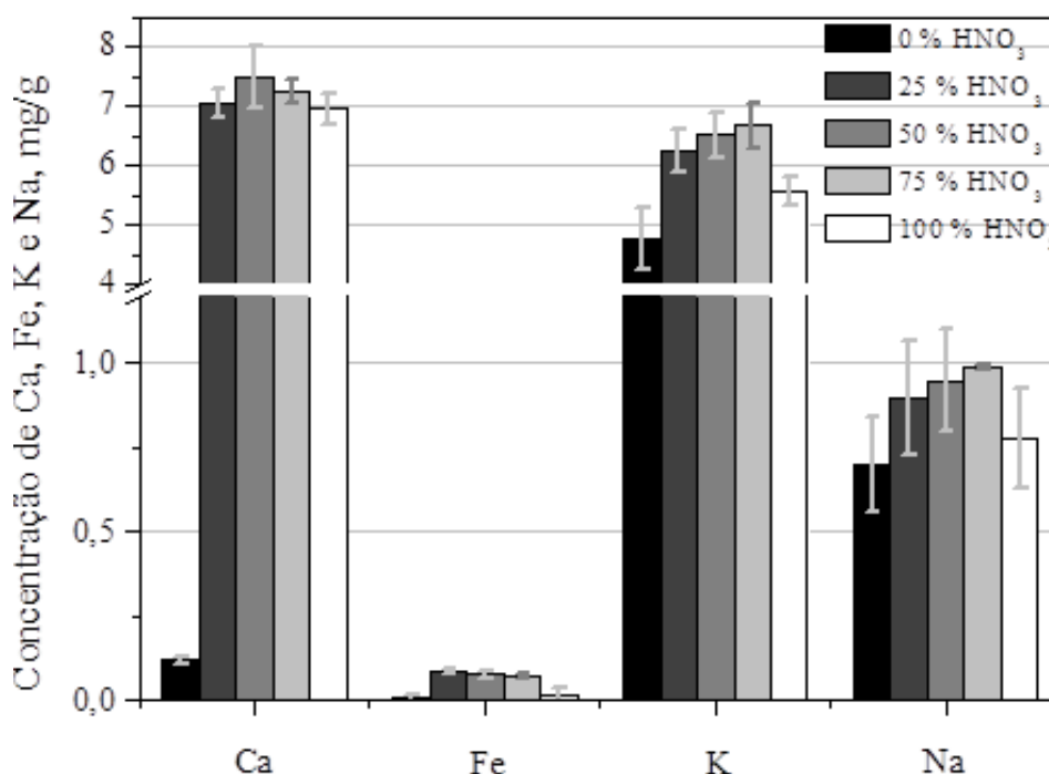
Figura 1. - Influência da concentração de ácido extrator sob a concentração de Ca, Fe, K e Na em achocolatado em pó. Tempo de extração de 30 min, temperatura de extração 50 \pm 5 °C. (média \pm intervalo de confiança 95%).
