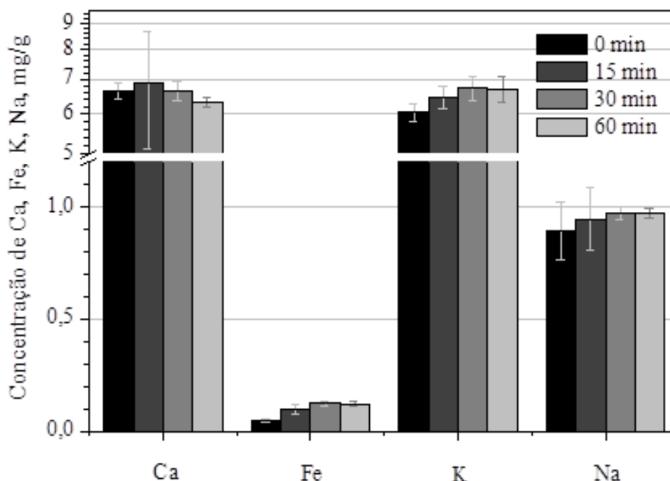
Figura 2. - Influência do tempo ação do ultrassom sob a concentração de Ca, Fe, K e Na em achocolatado em pó. Solução extratora de \text{HNO}_3 50% v/v, e temperatura de 50 \pm 5 °C. (média \pm intervalo de confiança 95%).
