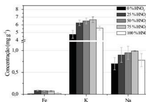
Figura 1. Influência da concentração de ácido extrator sob a concentração de Fe, K e Na em achocolatado empó. Tempo de extração de 30 minutos e temperatura de extração 50 \pm 5 °C. Resultados expressos como média \pm desvio padrão.
