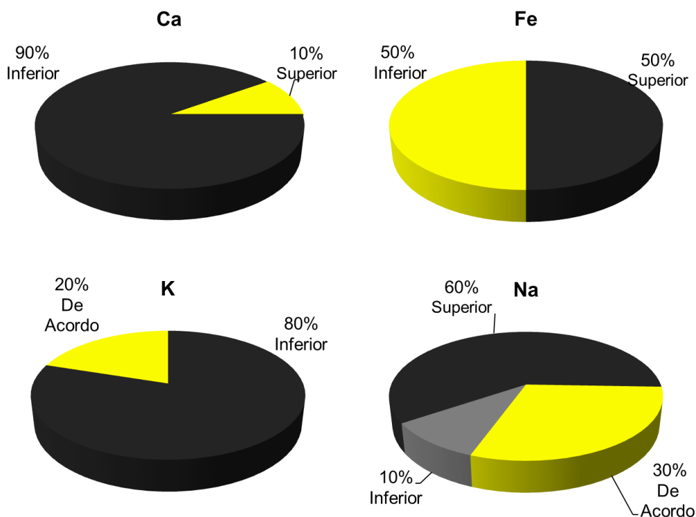
Figura 3. - Comparação das concentrações obtidas para Ca, Fe, K e Na em amostras de achocolatado em pó com os valores especificados na tabela TACO. Considerados os valores médios obtidos.
