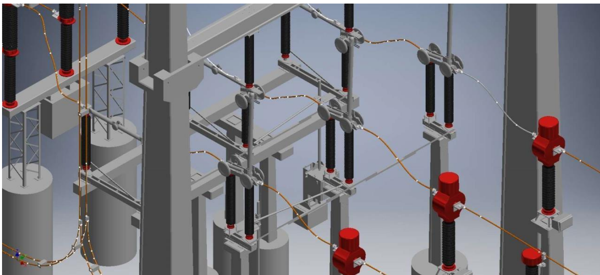
Figura 3: Ampliação do arranjo eletromecânico e fundações da SE Paranaíta
