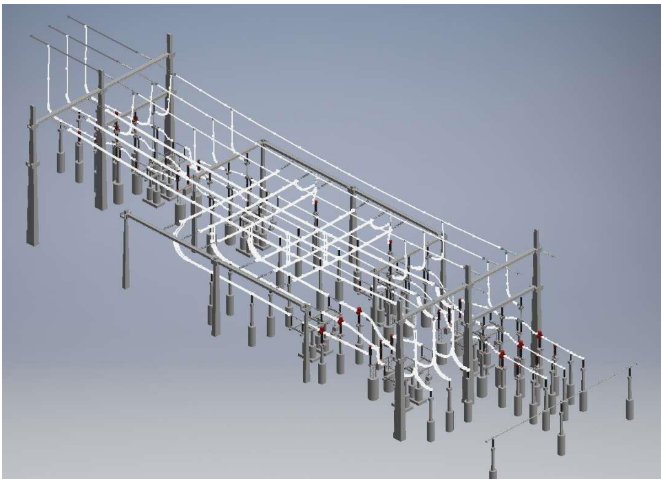
Figura 4: Maquete virtual do setor de 138 kV na SE Paranaíta 500/138 kV
