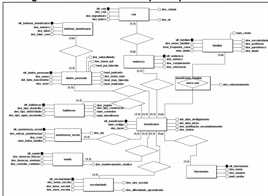
Figura 21 – DER do sistema para a primeira versão
