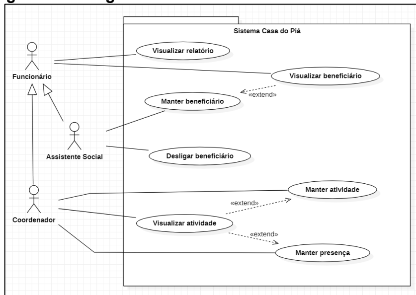
Figura 15 – Diagrama de Caso de Uso das funcionalidades
