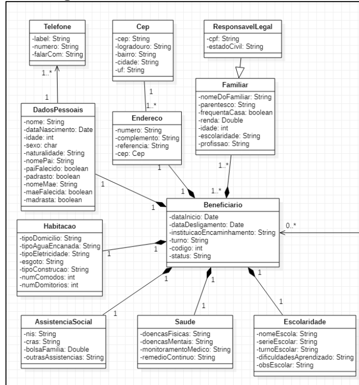
Figura 19 – Diagrama de classes da v1 focado no beneficiário
