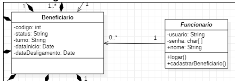
Figura 20 – Diagrama de classes da v1 focado no funcionário
