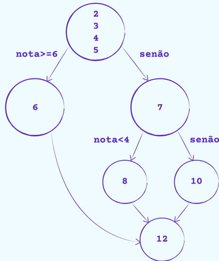
Figura 4 - Grafo de um se-senão encadeado
