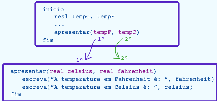
Figura 26 - Cuidado com a ordem dos argumentos
