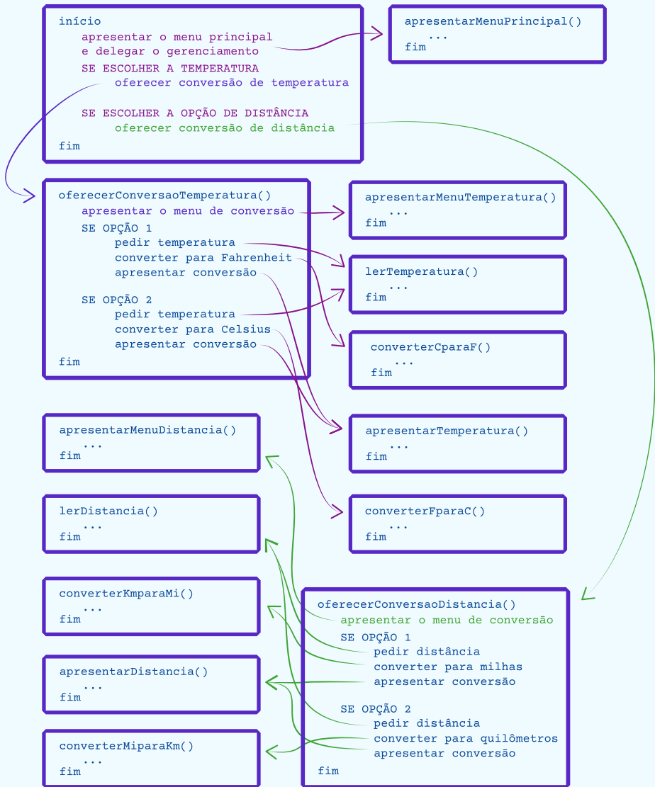
Figura 32 - Dividindo as responsabilidades das funções ainda mais
