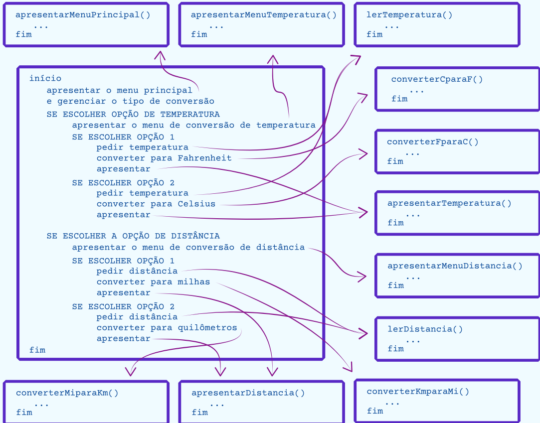
Figura 32 - Dividindo as responsabilidades das funções ainda mais
