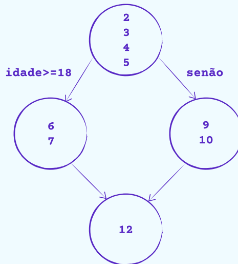
Figura 3 - Grafo de um se-senão
