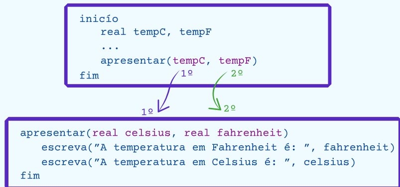
Figura 25 - Passagem de mais de um parâmetro
