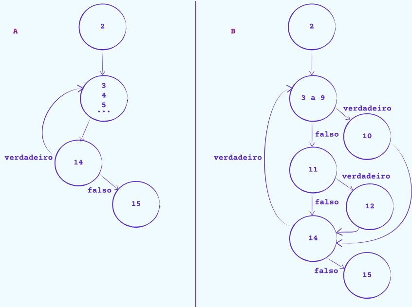
Figura 9 - Grafo do laço faça-enquanto
