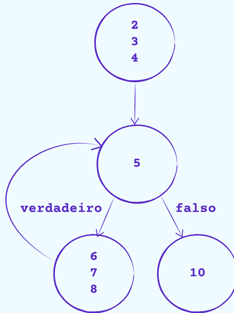
Figura 8 - Grafo do laço enquanto
