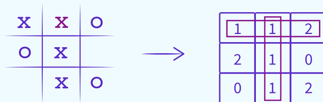
Figura 36 - Reduzindo verificações de vitória
