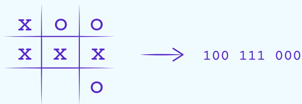
Figura 38 - Tabuleiro representado com 9 bits
