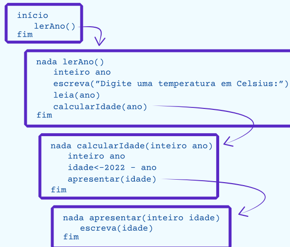
Figura 30 - Outra possível relação entre funções
