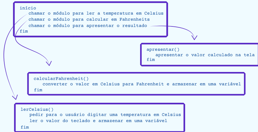
Figura 19 - Rascunhando funções
