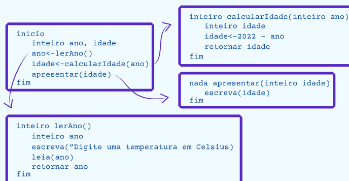
Figura 29 - Uma relação entre funções
