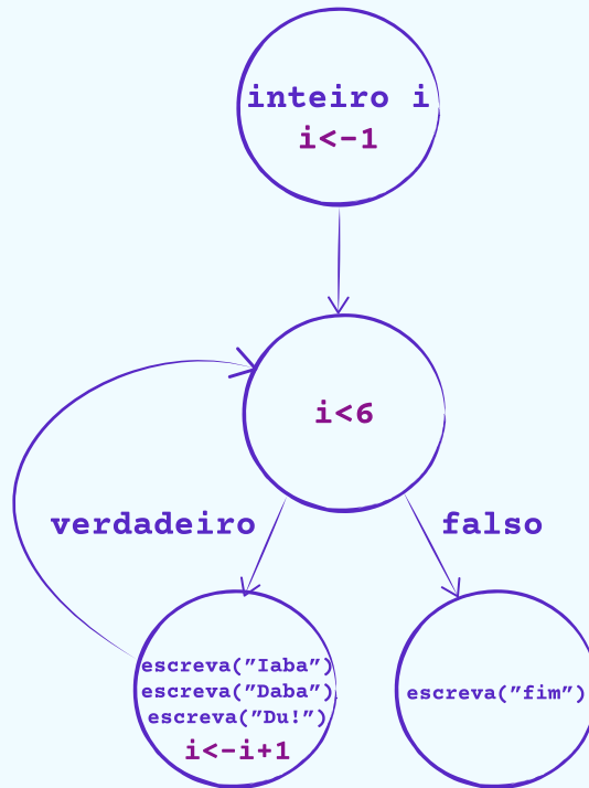
Figura 7 - Grafo do laço para
