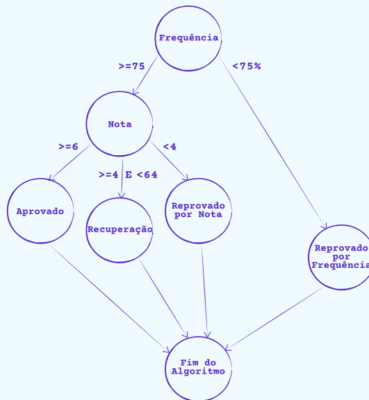
Figura 5 - se-senão aninhado
