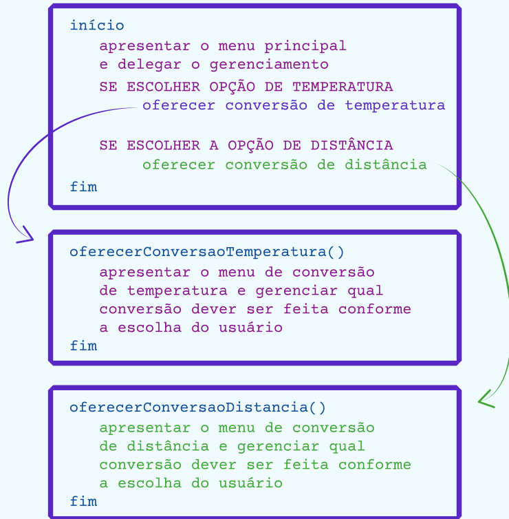
Figura 31 - Dividindo responsabilidades
