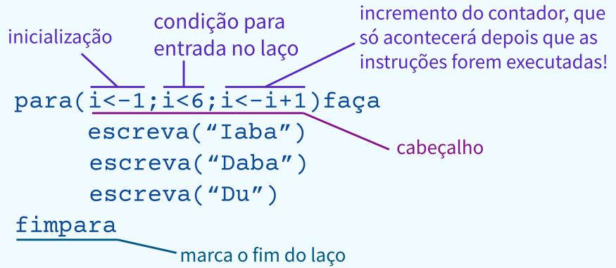
Figura 6 - Laço para
