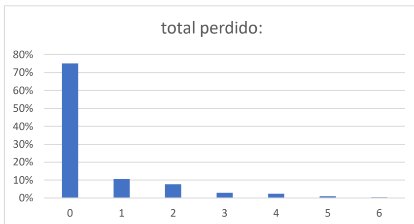
Teste 12d: Pacotes perdidos entre mensagens total
