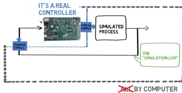
Figura 2 Processo Hardware-in-loop com Hardware Fonte: YouTube
