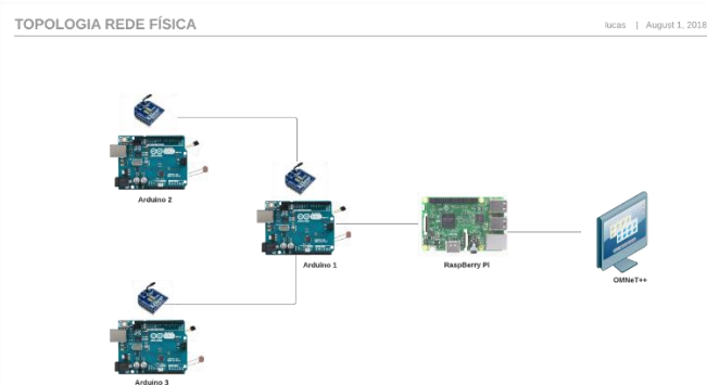
Figura 24 Topologia física
