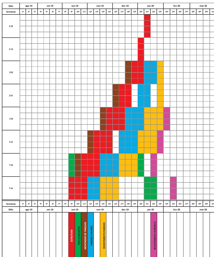
Figura 6 - Linha de balanço da obra versão final Fonte: o autor
