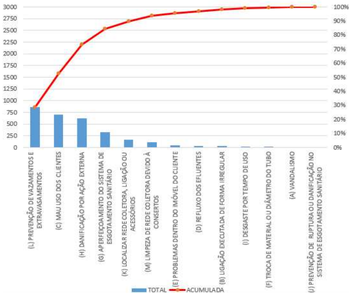
Figura 15 – Diagrama de Pareto dos motivos das manutenções preventivas e corretivas
