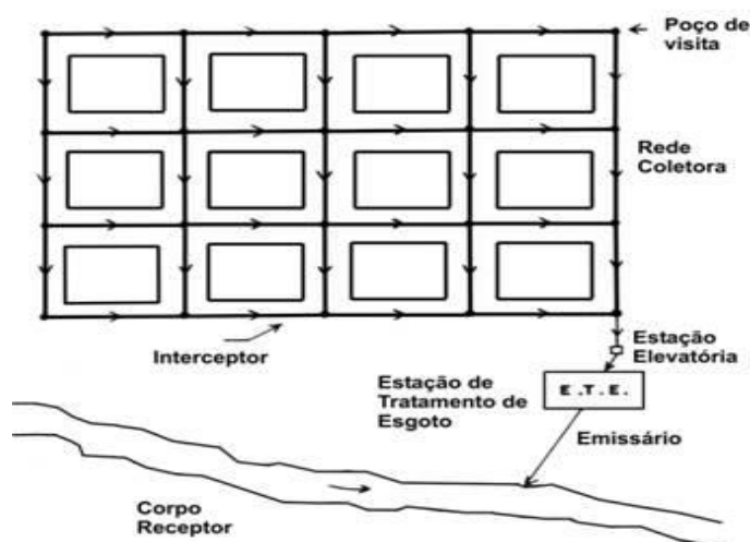
Figura 01 – Componentes de um sistema de esgotamento sanitário
